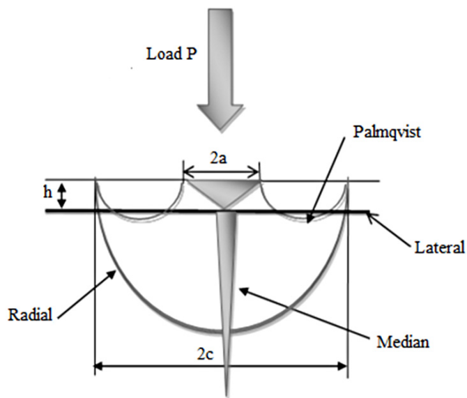
Fig. 3. Représentation schématisée des systèmes de fissures induits par indentation Vickers.
