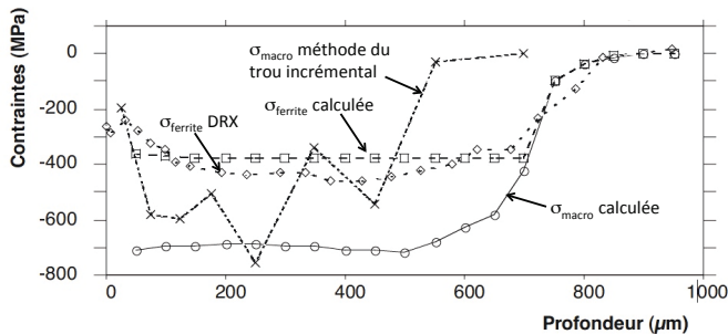
FIGURE 7. Comparaison entre les contraintes résiduelles macroscopiques (simulation et méthode du trou incrémental) et les contraintes résiduelles dans la ferrite (simulation et méthode par diffraction des rayons X [5]).
