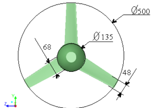
Fig. 2. Geometric parameters of the Rutland 503 rotor.
