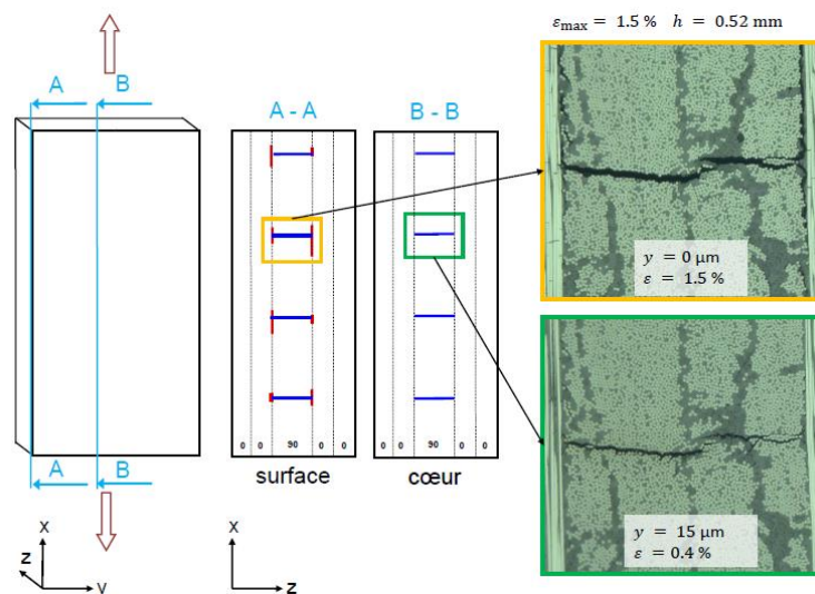
Figure 3 : Observations en surface et à cœur : schéma des sections observées et micrographies à la surface initiale ( y = 0\ \mu\text{m} ) et après abrasion ( y = 15\ \mu\text{m} ), stratification : [0_2/90_2/0_2]
