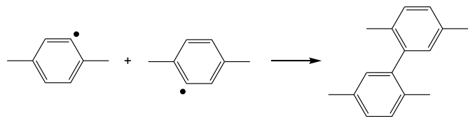
Fig. 20. Mécanisme de réticulation du PEEK par couplage intermoléculaire des radicaux phényle [3–6].
