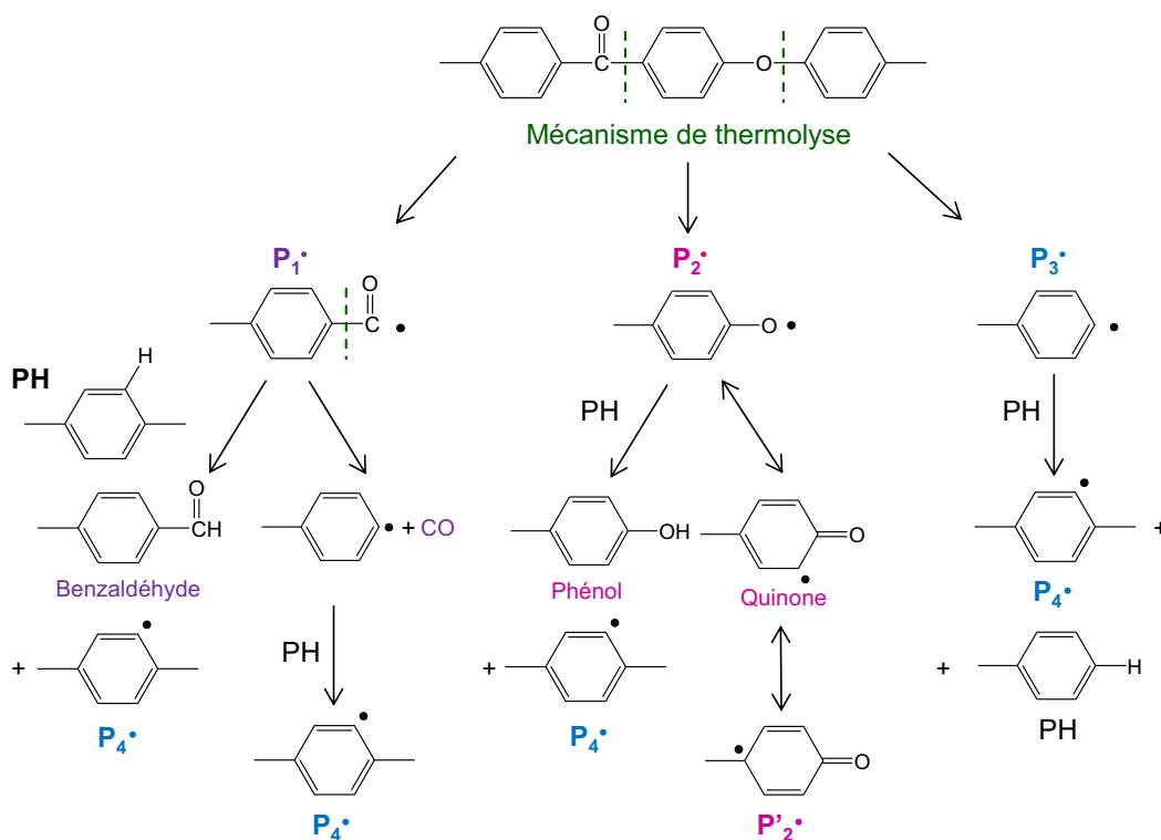
Fig. 11. Amorçage de la dégradation thermique du PEEK par rupture thermolytique de liaisons cétone et éther de la chaîne macromoléculaire. Formation de plusieurs espèces radicalaires notées : P_1^\bullet , P_2^\bullet , P_3^\bullet et P_4^\bullet .
