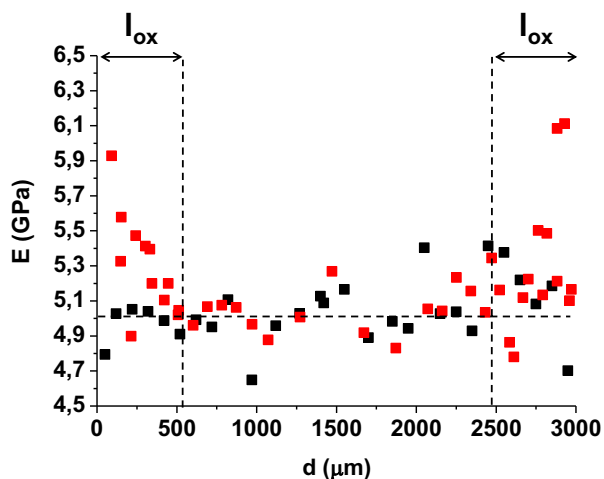
Fig. 15. Profil de module d'Young dans l'épaisseur d'une palquette de PEI avant (en noir) et après (rouge) 1966 h d'exposition dans l'air à 250 °C.
