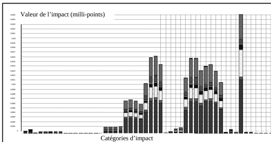
Figure 6. Résultats de l'ACV de la frégate La Fayette, pour la phase de construction et par la méthode de calcul d'impact CML 2001. Les différentes nuances de gris représentent les différents systèmes du navire. Les deux qui impactent le plus sont les systèmes flotteur et mobilité.
