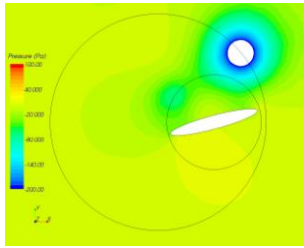
Fig. 17. contours de pression, \theta=0 degré, a15i
