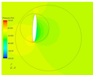
Fig. 19. contours de pression, \theta=144 degrés, a15i
