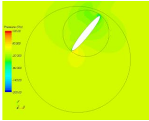
Fig. 18. contours de pression, \theta=72 degrés, a15i
