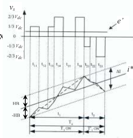
Figure A1. Représentation de la tension en sortie de l'onduleur et le courant dans cycle de modulation tirée de (Bose, 1990)
