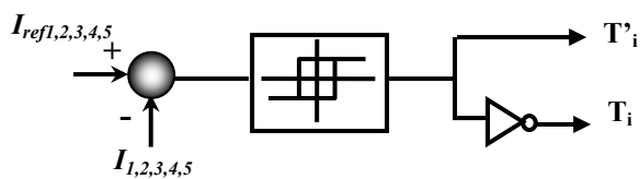
Figure 8. Schéma de la régulation du courant par hystérésis à bande fixe dans la base naturelle
