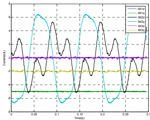
Fig. 6. dq currents in Fault Mode (Experimental Results)
