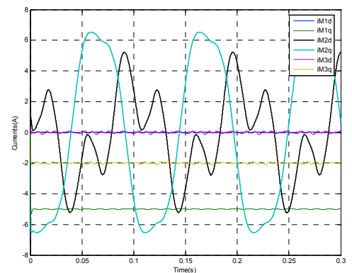
Fig. 9. dq currents in Fault Mode (Simulation Results)
