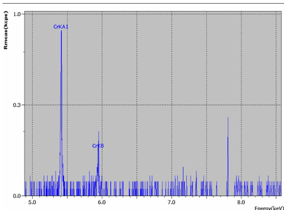
Figure 1. Analyse par fluorescence X d'une couche de chrome.
