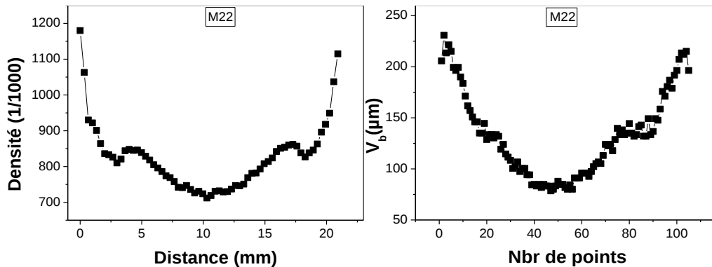
Figure.7. Corrélation entre le profil de la densité et celui de l'usure en dépouille V_b .
