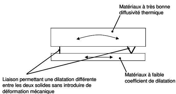
Fig. 12. – Exemple de liaison rigide en flexion et laissant libre la dilatation longitudinale.
