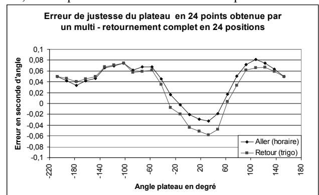
Figure 7 : Erreur de justesse du plateau sur un tour
