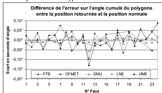
Figure 9 : Cohérence en position normale et retournée
