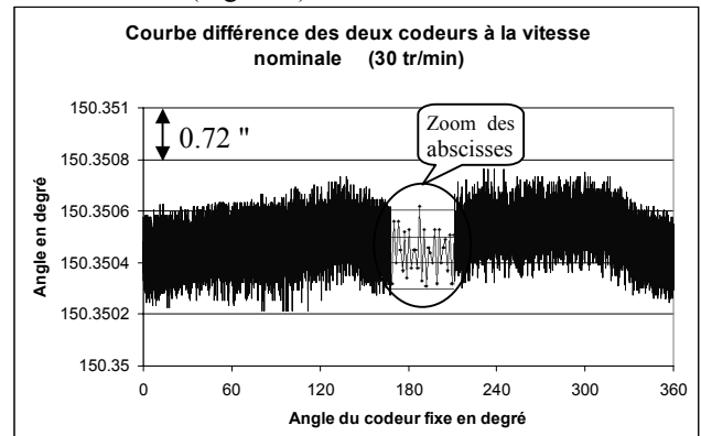
Figure 5 : Sous échantillonnage des lectures codeurs
