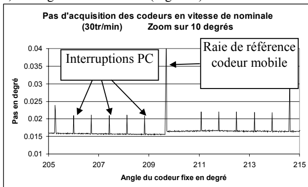
Figure 4 : Pas d'acquisition du système de mesure
