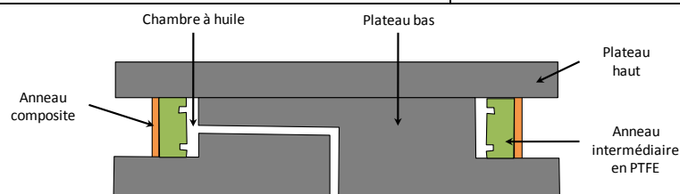
Figure 6 : Dispositif de mise sous pression interne d'un anneau d'après [Cain et al, 2009]
