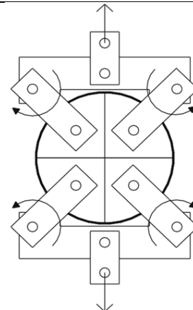
Figure 5 : Montage pour l'essai avec des quarts de disques [Walsh, 2008]
