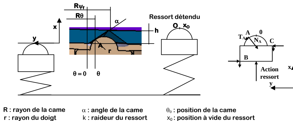
FIG. 7 – Evolution du doigt durant la fermeture et actions de contact.
