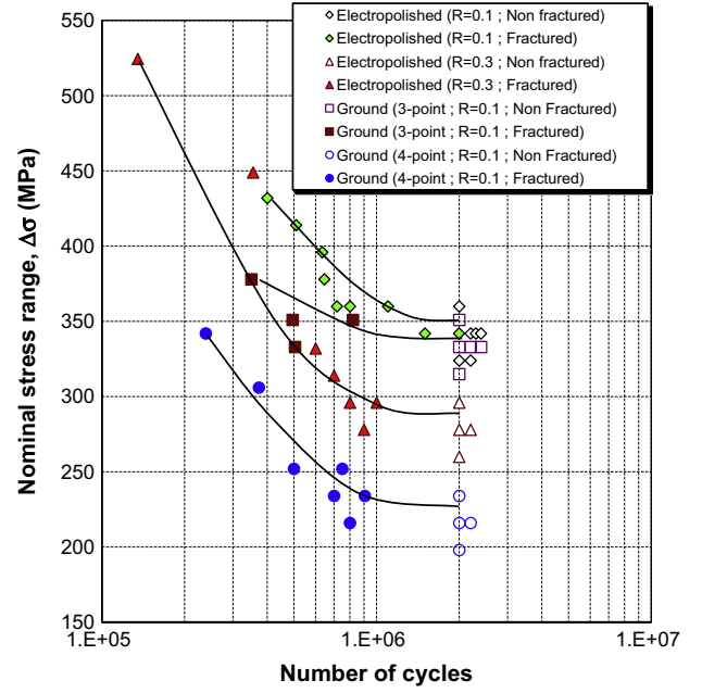
Fig. 7. SN diagram.
