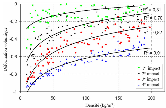
Fig. 12. Évolution de la déformation volumique des grains en fonction de leurs densités et à différentes étapes de la compression dynamique.
