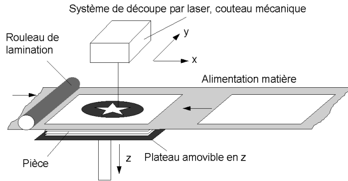
Figure 10 : principe de la fabrication par découpe et collage de strates
