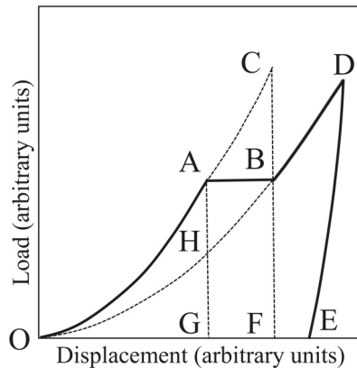
Fig. 4. Courbe d'indentation en charge imposée montrant le déplacement brutal de l'indenteur causé par l'écaillage du film. Les lettres A à H délimitent les domaines utilisés pour calculer l'énergie de fissuration.
