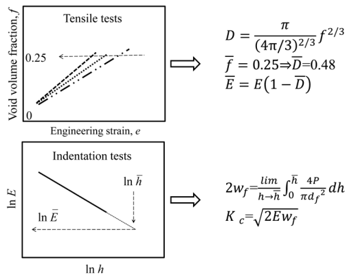
Fig. 7. Méthode de Lee et al. [101] pour le calcul de la ténacité : a- détermination de la fraction volumique de cavités correspondant à l'initiation de la fissure. b- Cette valeur est fixée à 0,25, ce qui correspond à un dommage de 0,48. c- En représentation bilogarithmique, le module d'Young mesuré par indentation varie linéairement en fonction de la profondeur indentée. Cette courbe est extrapolée pour les plus grandes profondeurs de pénétration et le module d'Young critique ( \bar{E} = 0,48E ) permet de trouver la profondeur critique d'indentation correspondante. d- La profondeur critique est la borne supérieure de l'intégrale permettant de calculer l'énergie de rupture puis la ténacité.
