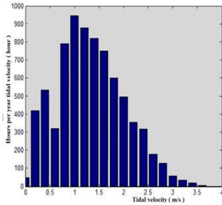
Fig. 13: Raz de Sein site tidal histogram
