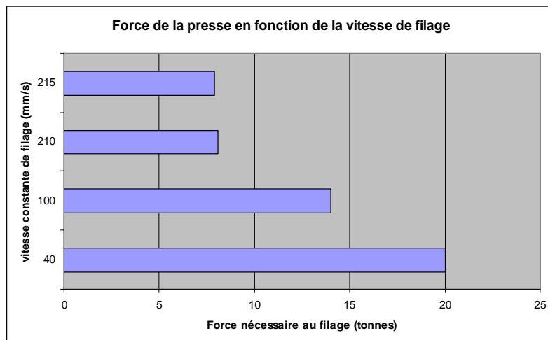
Figure 4 – Effort obtenu en fonction de la vitesse du coulisseau
