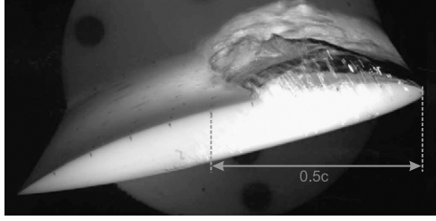
(d) \alpha^+ = 14.5^\circ .
