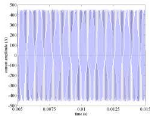
Figure 11. Courant dans la machine homopolaire, MLI intersective
