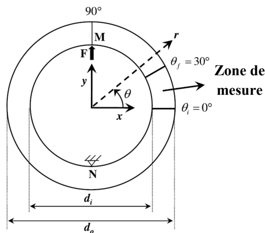
FIGURE 4 – Zone de mesure utile pour l'identification des propriétés mécaniques.
