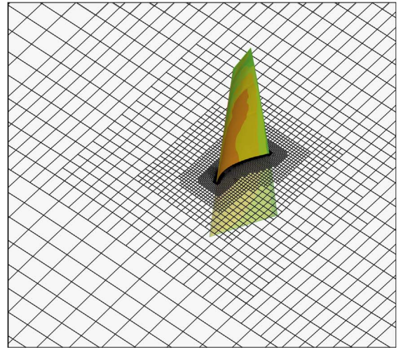
(d) Mesh of S_{Remesh} after remeshing S_{Def} .
