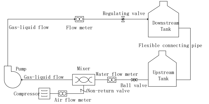
Fig. 1. Test rig
