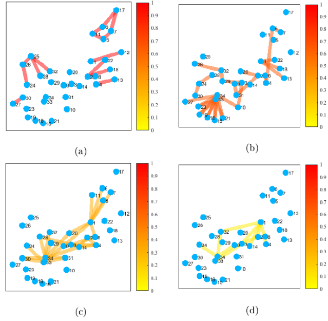
FIGURE 4 – (a) Niveau 1 de vulnérabilité pour le réseau Karate club (b) Niveau 2 de vulnérabilité (c) Niveau 3 de vulnérabilité (d) Niveau 4 de vulnérabilité.
