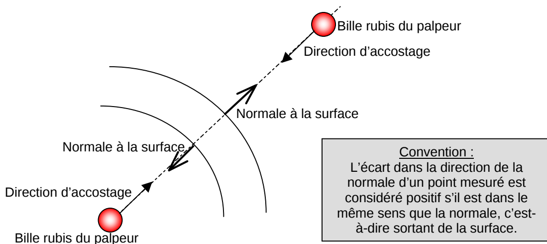
Figure III : Schéma explicatif du palpage dans la direction des normales et du signe des écarts
