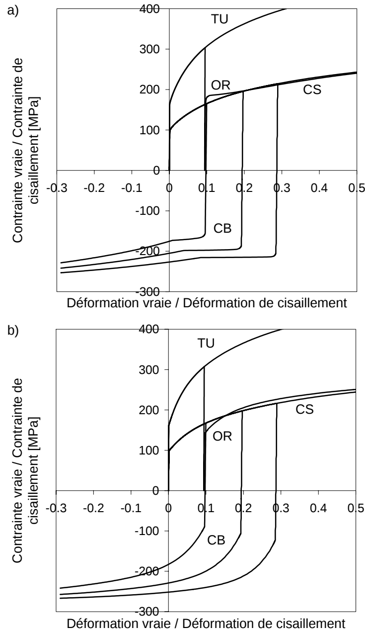
Figure 1. Prédictions rhéologiques avec a) le modèle microstructural de Teodosiu et Hu et b) le modèle classique de Chaboche. TU: traction uniaxiale ; CS: cisaillement simple; BS: cisaillement Bauschinger à 10, 20 et 30% de pré-déformation ; OR: traction uniaxiale à 10% de pré-déformation suivie d'un cisaillement simple dans la même direction.
