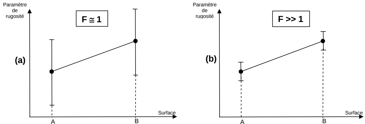
Figure 4. Illustration des cas possibles et incidence sur l'analyse de la variance
