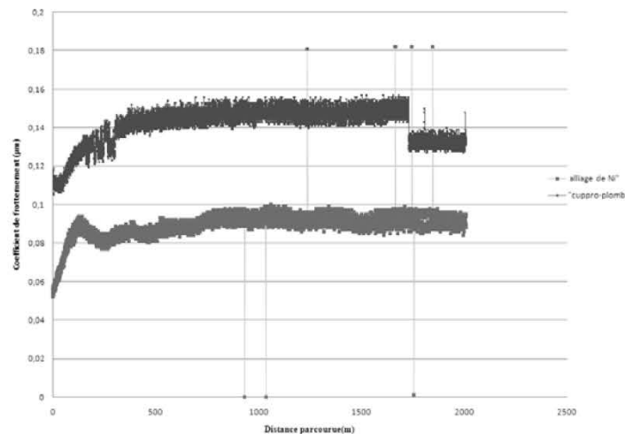
Figure 1 : Courbes expérimentales de l'évolution du coefficient de frottement en fonction de la distance parcourue de l'alliage de Ni et du cuppro-plomb sous charge de 12N et vitesses 50 mm s-1.
