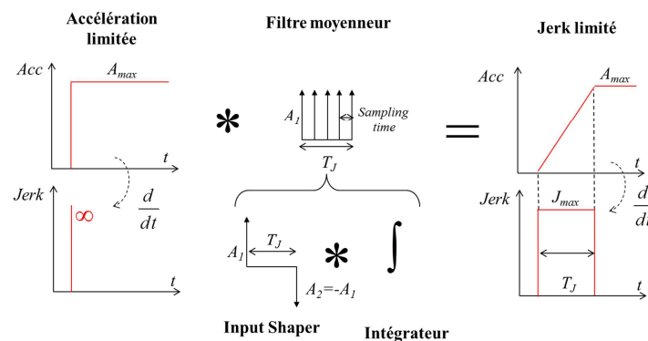
Fig. 7 : Filtrage équivalent pour synthèse d'une trajectoire à jerk limité.
