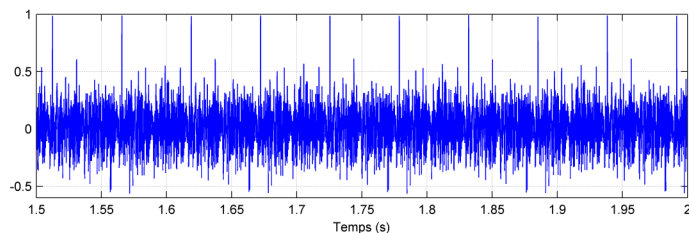
FIGURE 4 – Identification de l'émetteur par corrélation.
