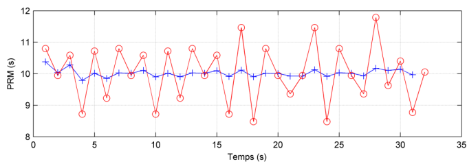
FIGURE 6 – PRM réelles (rouge), PRM estimées (bleu).
