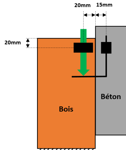
Figure 3: Placement des capteurs de déplacements sur les corps d'épreuve
