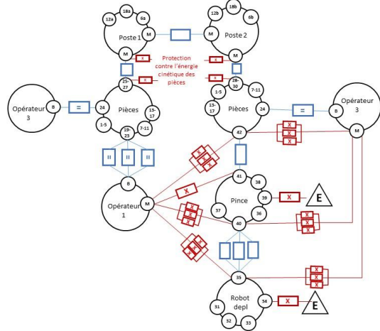
Figure 7 : Modèle énergétique simplifié pour la phase de production avec un robot
