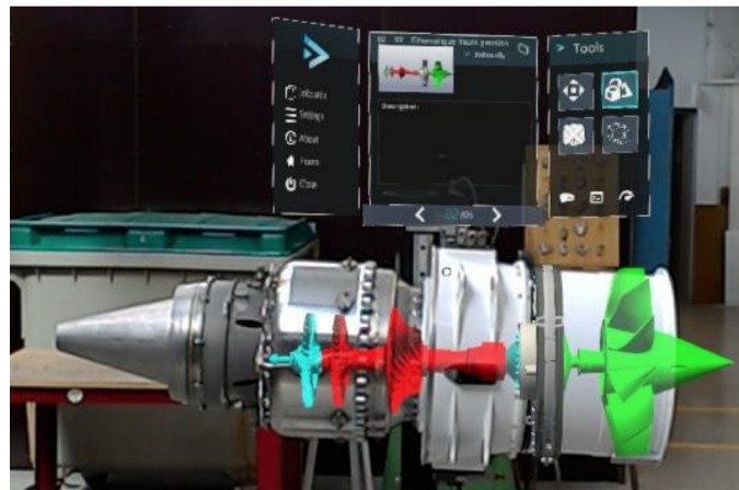
Figure 14. AR Hololens turbofan scenario.
