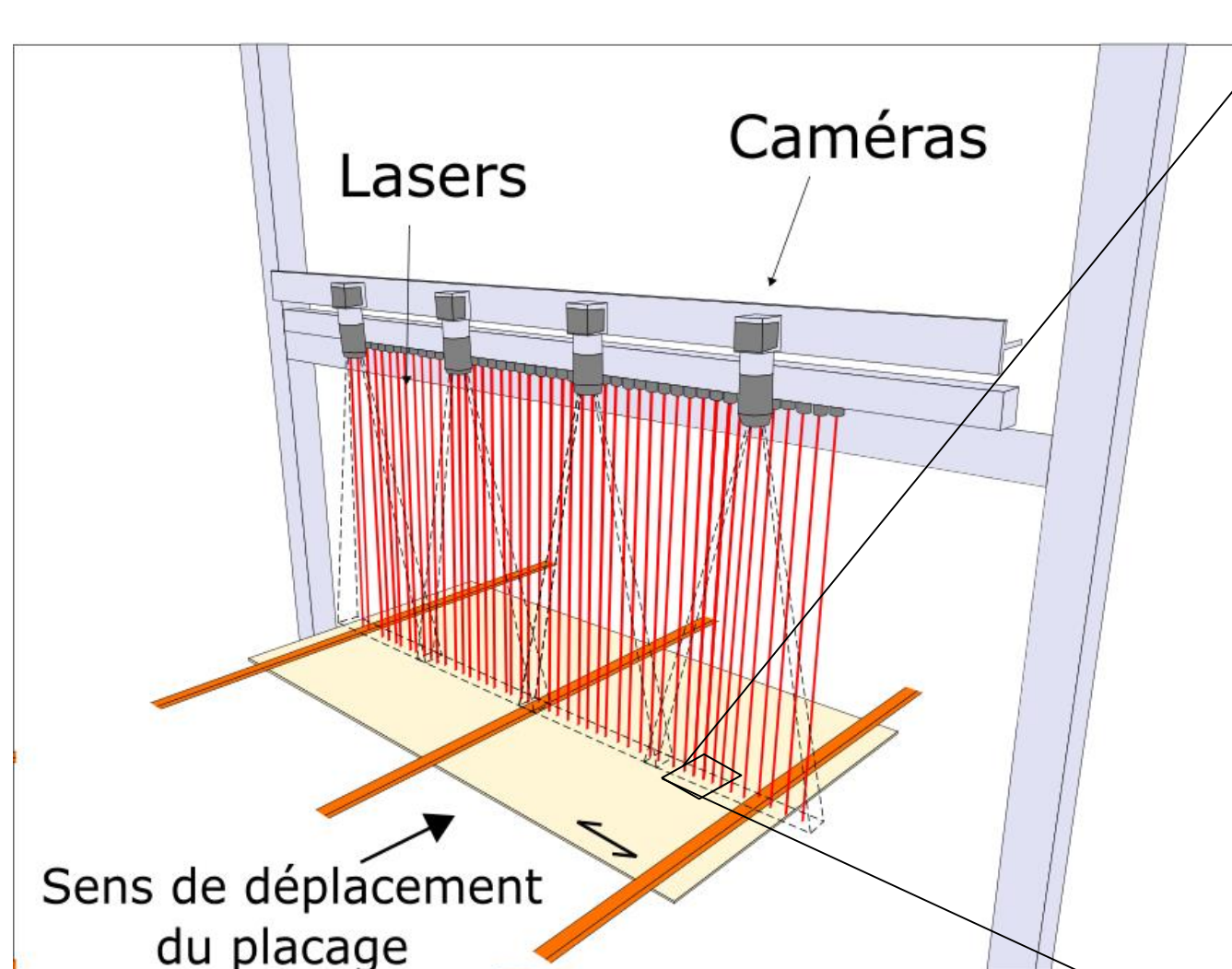
Matériel optique de FEMTO - ST Chaîne de déroulage du LaBoMaP (à droite), et le schéma de la ligne de lasers (à gauche)
