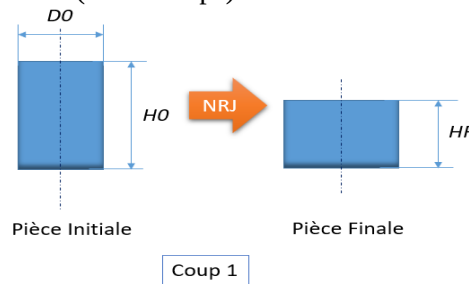
Figure 3. Schéma du refoulement simple pour un (1) coup.
