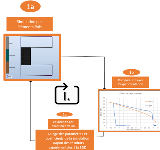
Figure 7. Le modèle éléments finis.
