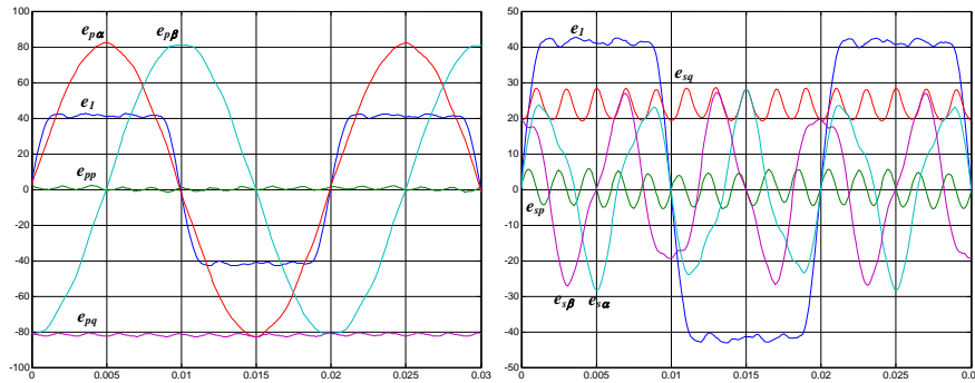
Figure 5.15. Forces électromotrices des machines principales et secondaires avant ( e_{\alpha\beta} ) et après rotation ( e_{dq} ) comparées à la force électromotrice de la phase 1 ( e_l )
