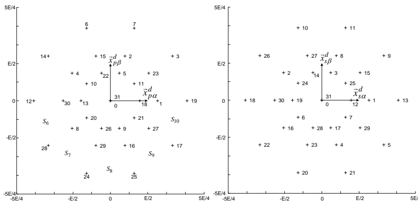
Figure 5.7. Représentation graphique d'un onduleur pentaphasé dans les sous-espaces principal (à gauche) et secondaire (à droite)
