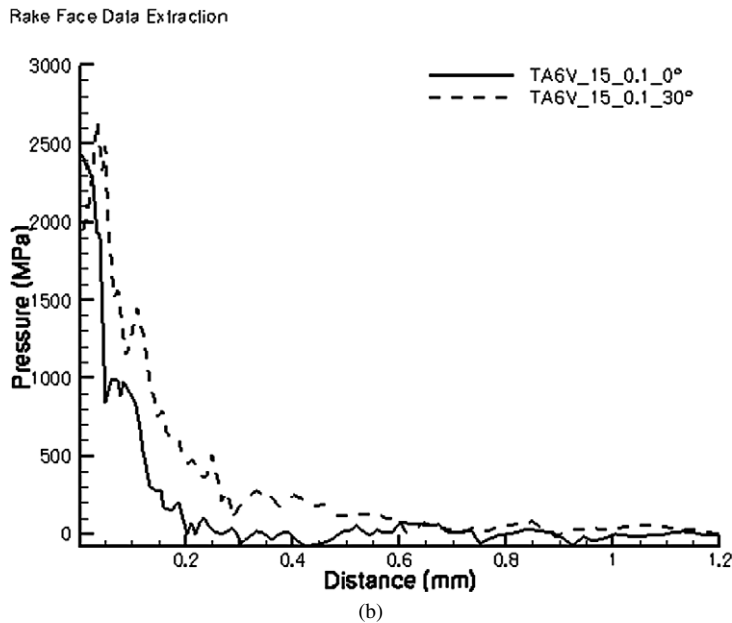
Fig. 7. Evolution des paramètres tribologiques pour deux géométries différentes 0^\circ et 30^\circ . La vitesse de coupe V_c = 15 m/min et l'avance f = 0.1 mm. (a) Température de coupe. (b) Pression de contact.
