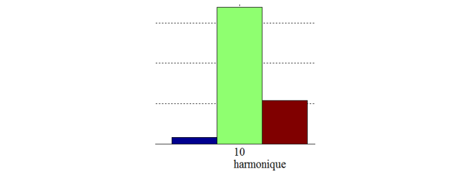
Figure 11 : Contenu harmonique du couple électromagnétique de la machine 20/8/5 (estimation analytique)
