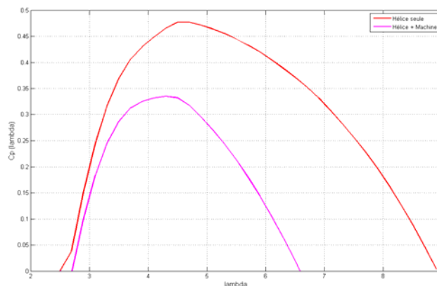
Figure 7: Résultats issus des modèles
