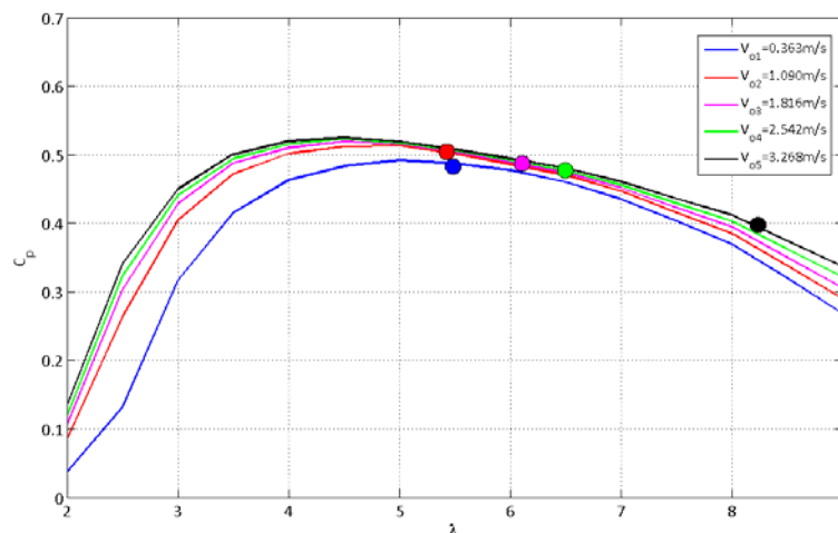
Figure 5: Points de fonctionnement dans un plan C_p(\lambda) (courbes de performance de l'hélice seule)
