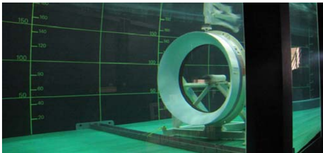
Figure 6 : Maquette académique en test et résultats d'essais
