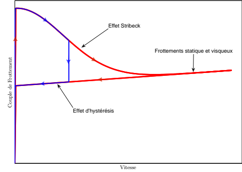
Fig. 3. Exemple de modèle de frottement avec hystérésis
