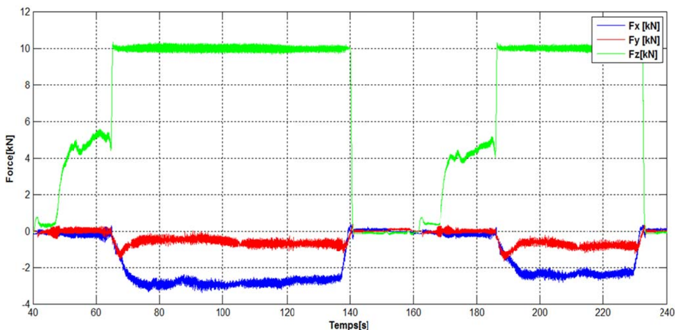
Figure 12 : Évolution des trois composantes d'effort lors des soudures circulaires fermées D2-1g et D2-1p, soudures réalisées successivement sans temps d'attente
