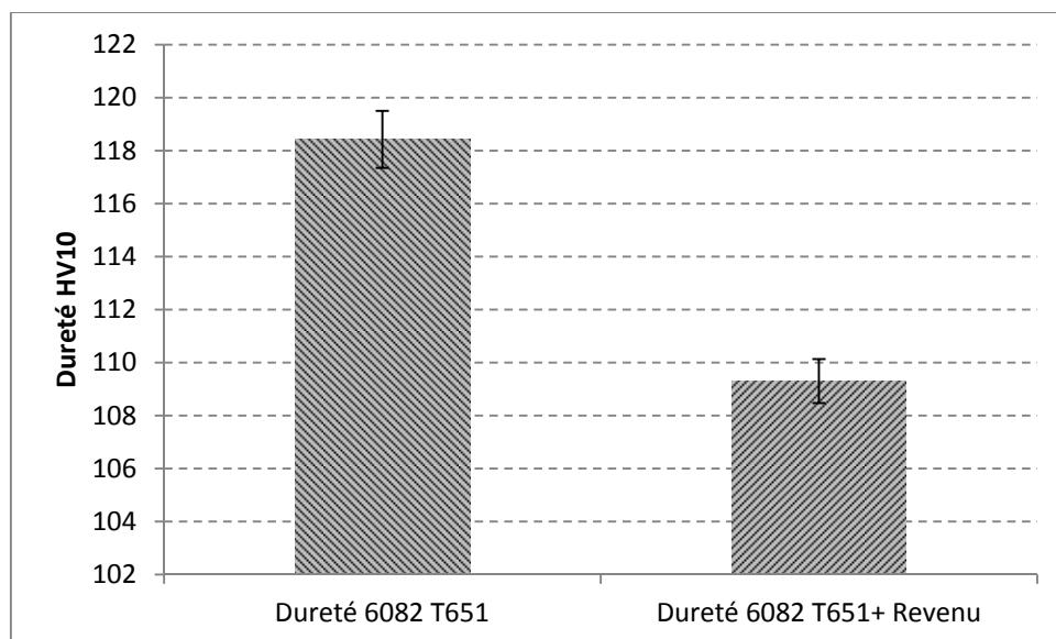
Figure 57 : Dureté moyenne des coupons à souder.
