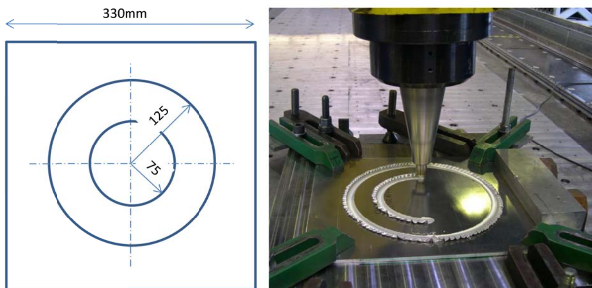
Figure 11 : Photographie du dispositif expérimental pour les soudures circulaires
