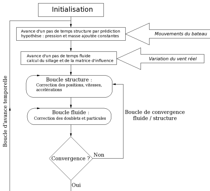
Figure 2. Schéma de couplage
