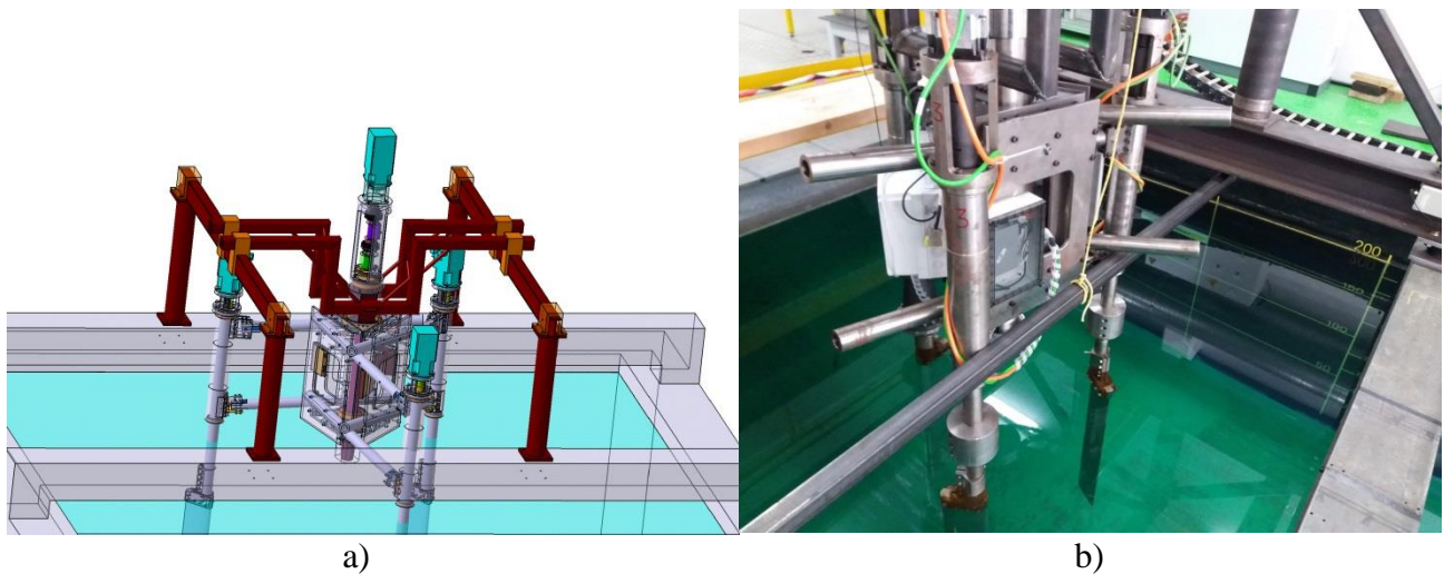
Figure 1. a) CAO de SHIVA ; b) SHIVA dans le bassin Ifremer de Boulogne-sur-Mer
