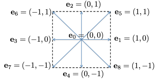
Fig. 4.1 D2Q9 lattice node
