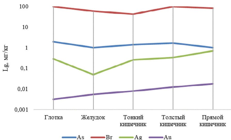
Рис. 2. Распределение Ag, Au, Br, As в пищеварительной системе свиньи домашней на территории г. Экибастуз, Лg (мг/кг) / Fig. 2. The distribution of chemical elements (Ag, Au, Br, As) in the digestive system of Sus scrofa domestica in the territory of Ekibastuz, Lg (mg/kg)
